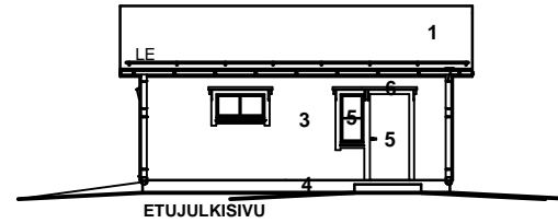
ETUJULKISIVU
